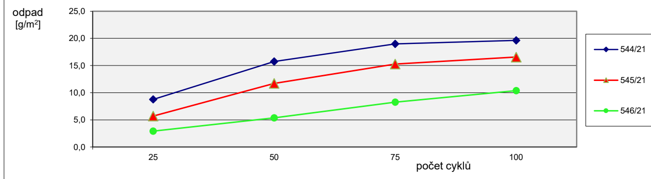
Průběh odpadů betonu
